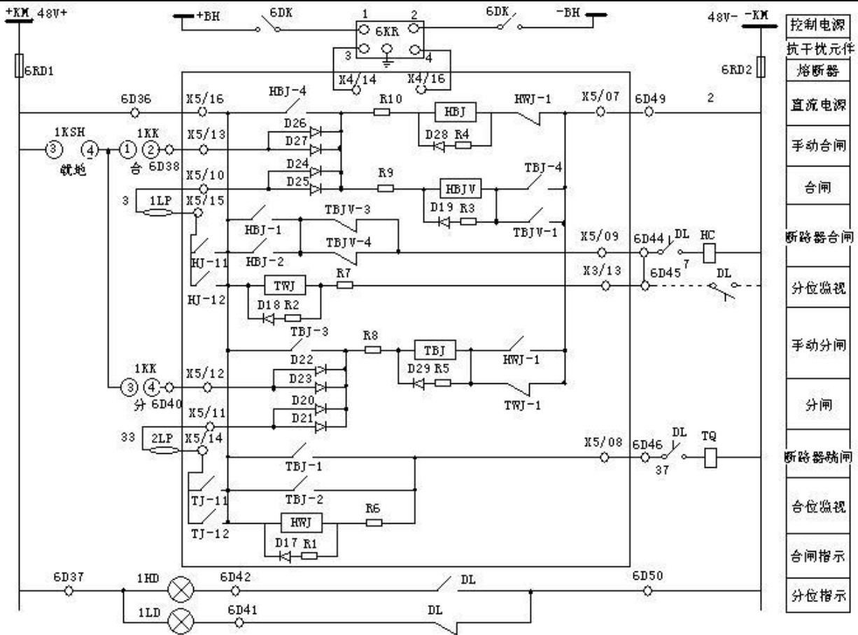
10kV 电容器保护装置原理图
